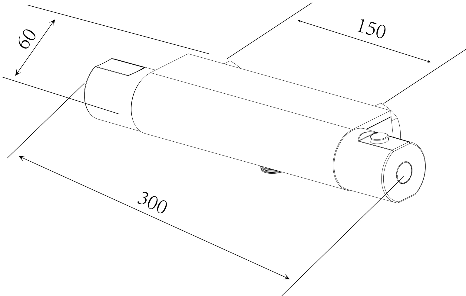
109566 沐浴龍頭尺寸圖
